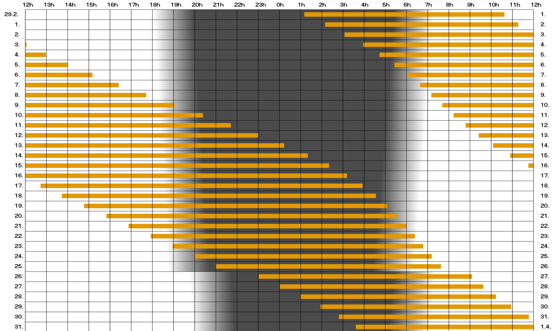
Sichtbarkeit des Mondes im März 2016 (berechnet für Boden)
